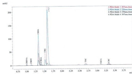
Cannabinoid Gehalt des erhaltenen Öles, in % der Gesamtmasse
